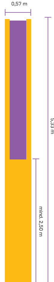
Seitenansicht
