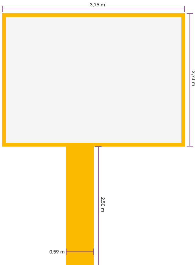
Frontansicht
