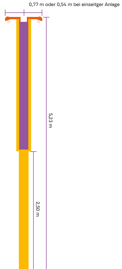
Seitenansicht
